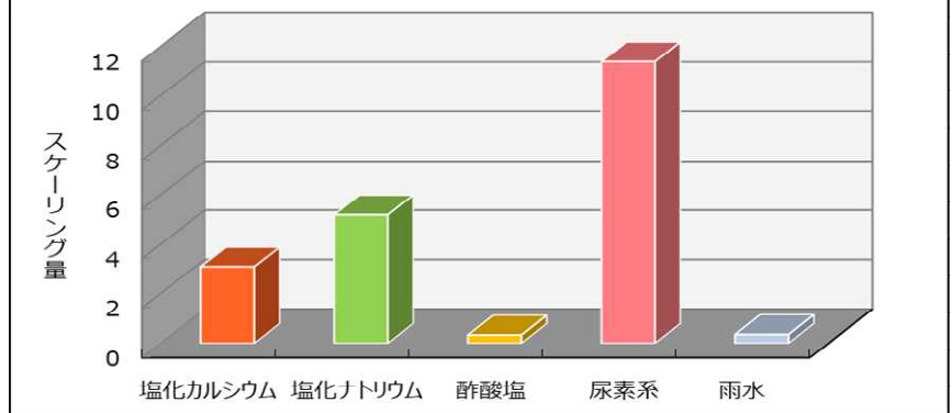
凍結融解試験によるコンクリート劣化
