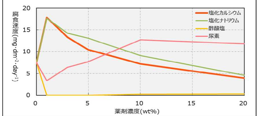
腐食速度と凍結防止剤濃度の関係*3
